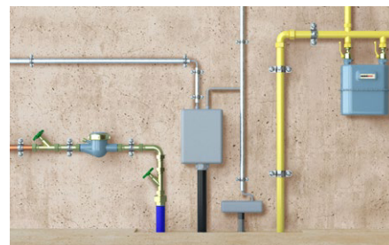
Fissaggio di tubi
